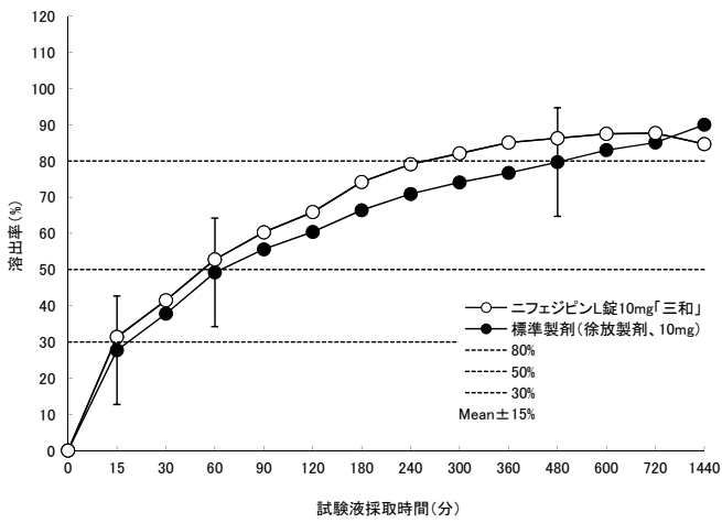
試験液:pH6.8
