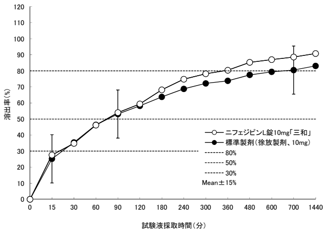
試験液:pH1.2
