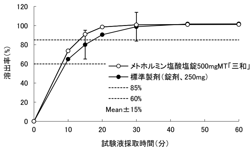
図 5 溶出挙動の比較（回転数：100rpm、試験液：pH1.2）
