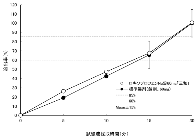
試験液:pH4.0 [判定基準:B]
