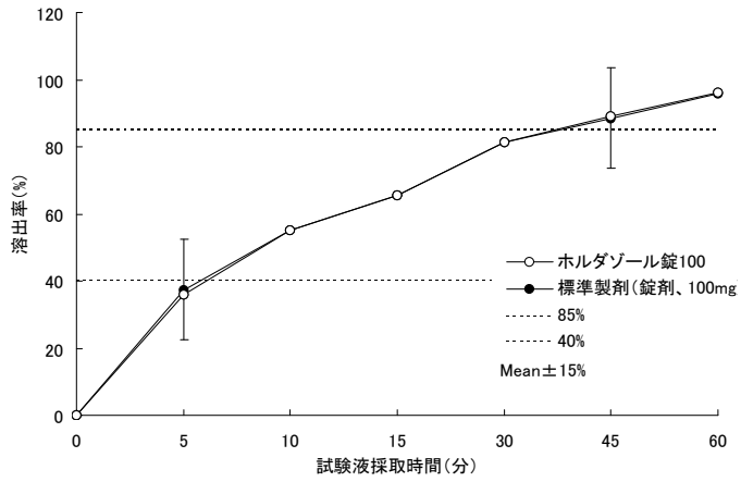
試験液: pH6.8 [判定基準C]
