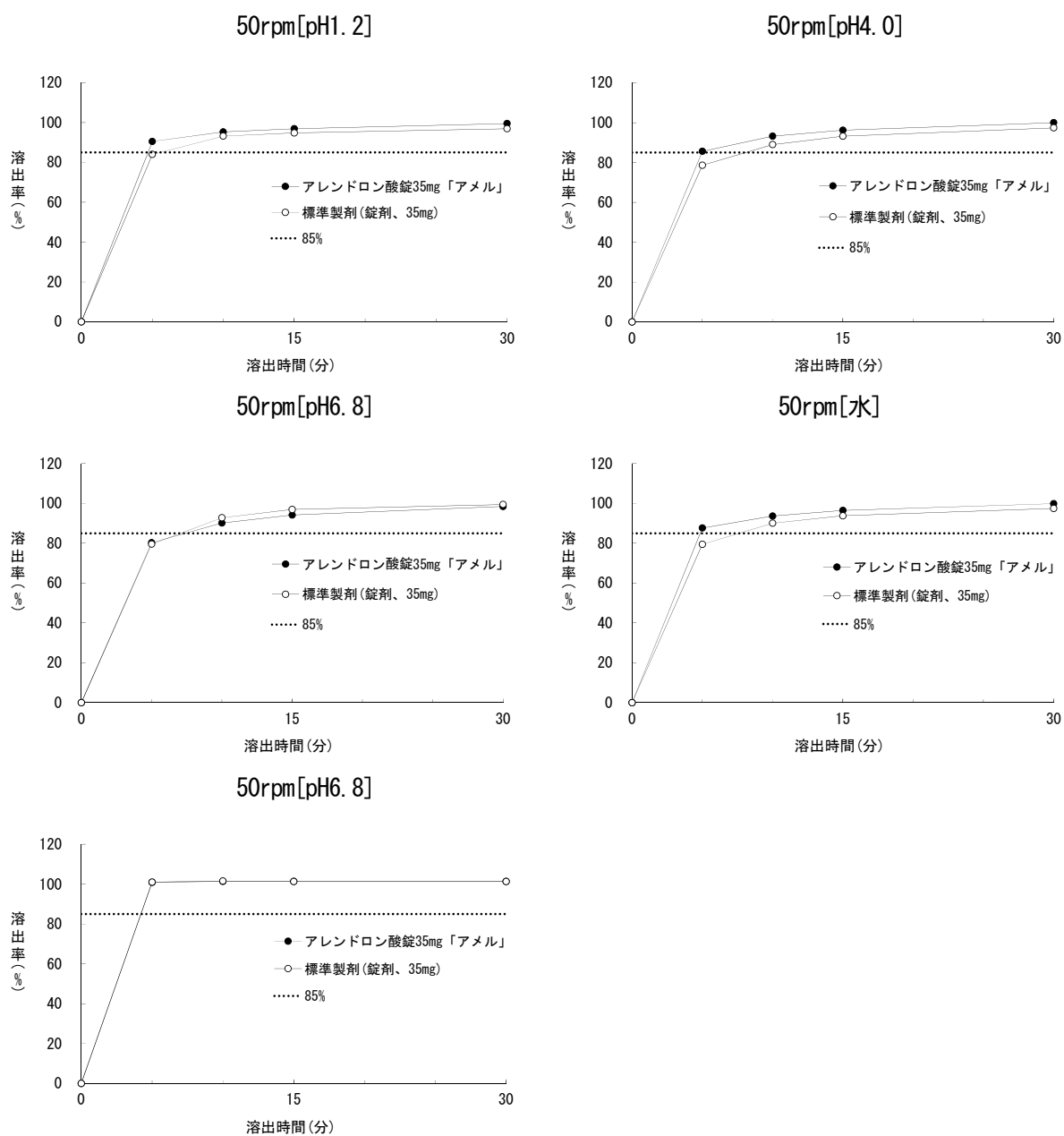
図. 溶出曲線
