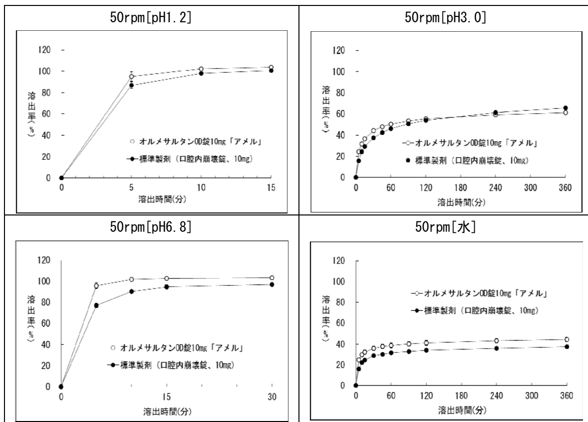
図 2. 溶出曲線
