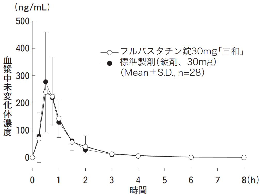
図 1 血漿中未変化体濃度推移
